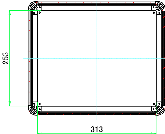
C-C ( 1 : 6 )
