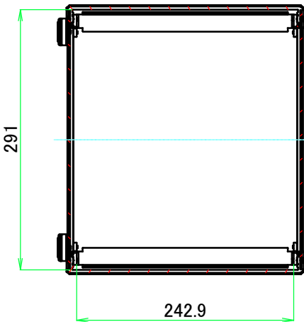
B-B ( 1 : 6 )
